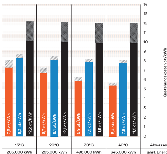
Gestehungskosten auf Lebensdauer bei 4,5m³/h Abwasser (Zieltemperatur 40°C)
